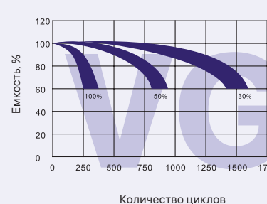
Влияние глубины разряда на циклический ресурс
