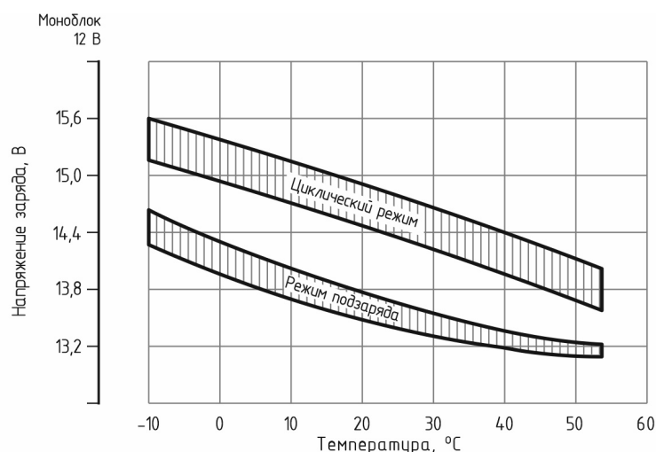
Рис. 4 - Соотношение между напряжением заряда и температурой
