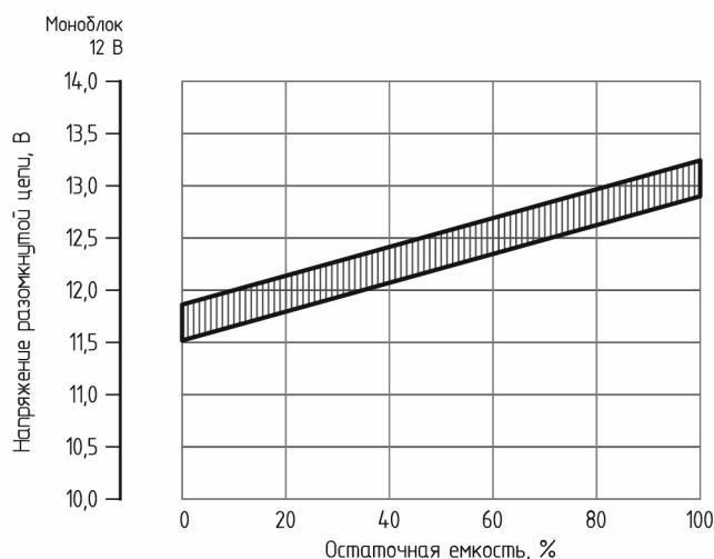
Рис.2 - Напряжение разомкнутой цепи аккумулятора в зависимости от остаточной емкости
